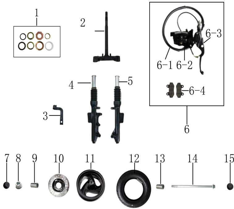
图3 下联板、左右前减、前轮泥板、前轮胎及前碟刹泵总成
