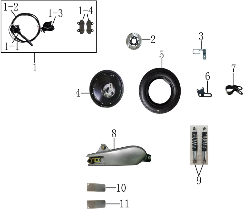
图6 后平叉、后减震、后轮胎、电机及后轮挡泥板
